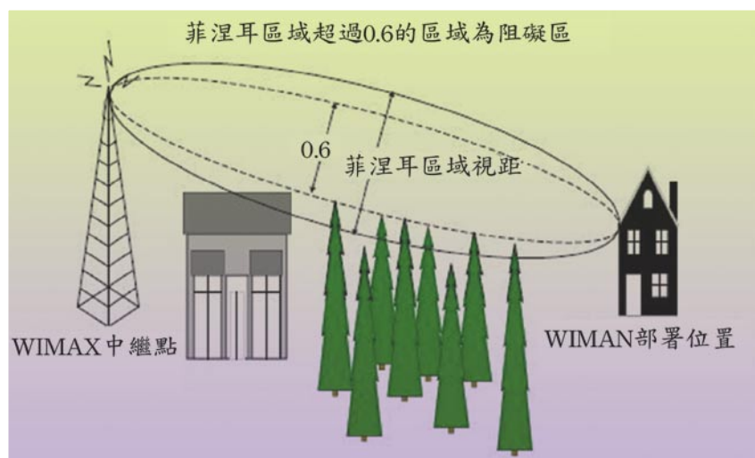
圖一 菲涅耳區域視距傳輸示意圖
