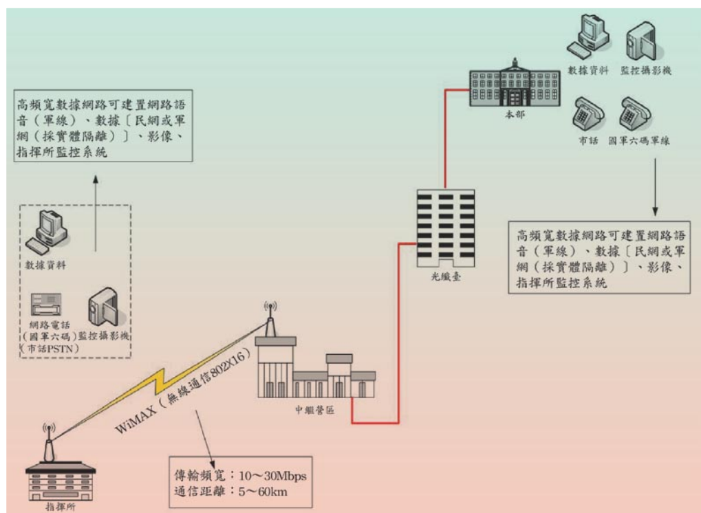
圖七 WiMAX結合中繼營區通信架構圖
