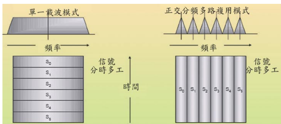
圖二 OFDMA單一載波模式、發送波形圖
