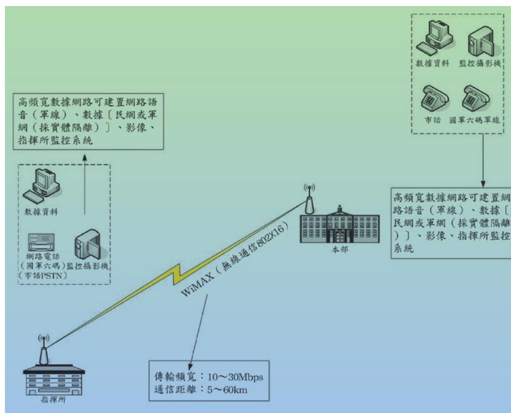
圖五 WiMAX通信架構圖
