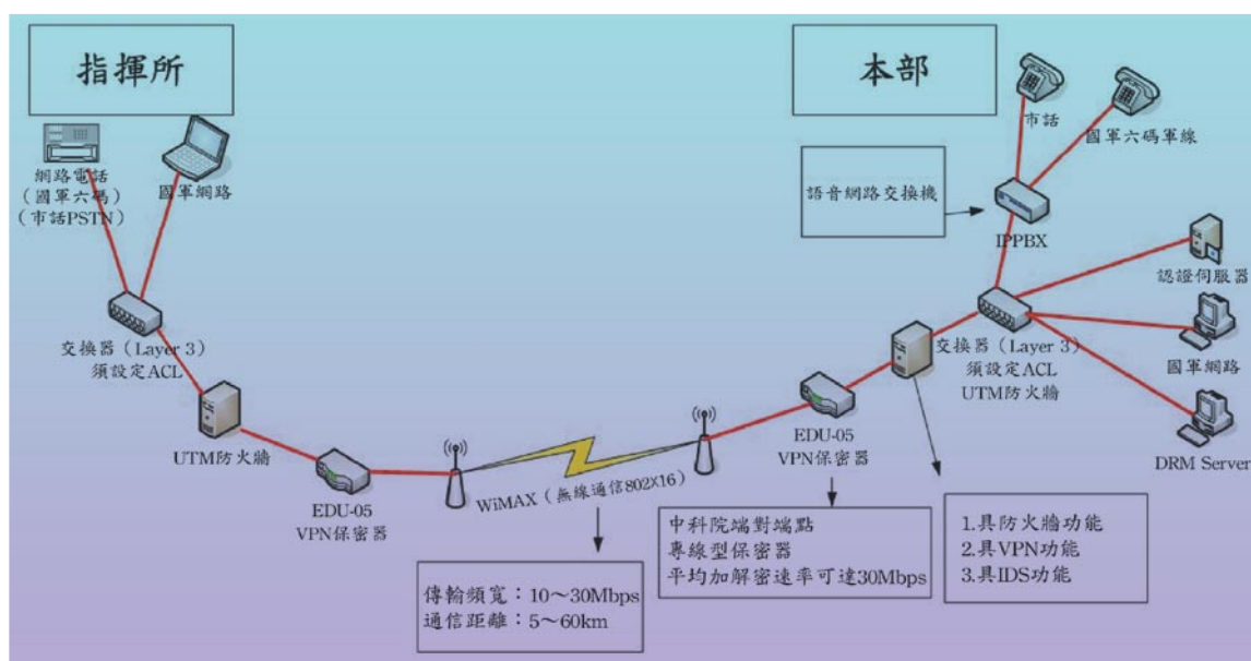
圖八 WiMAX網路安全構想圖（軍民網實體區隔）
