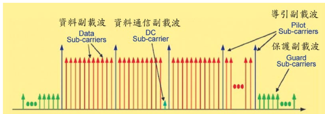
圖三 OFDMA子載波結構圖
