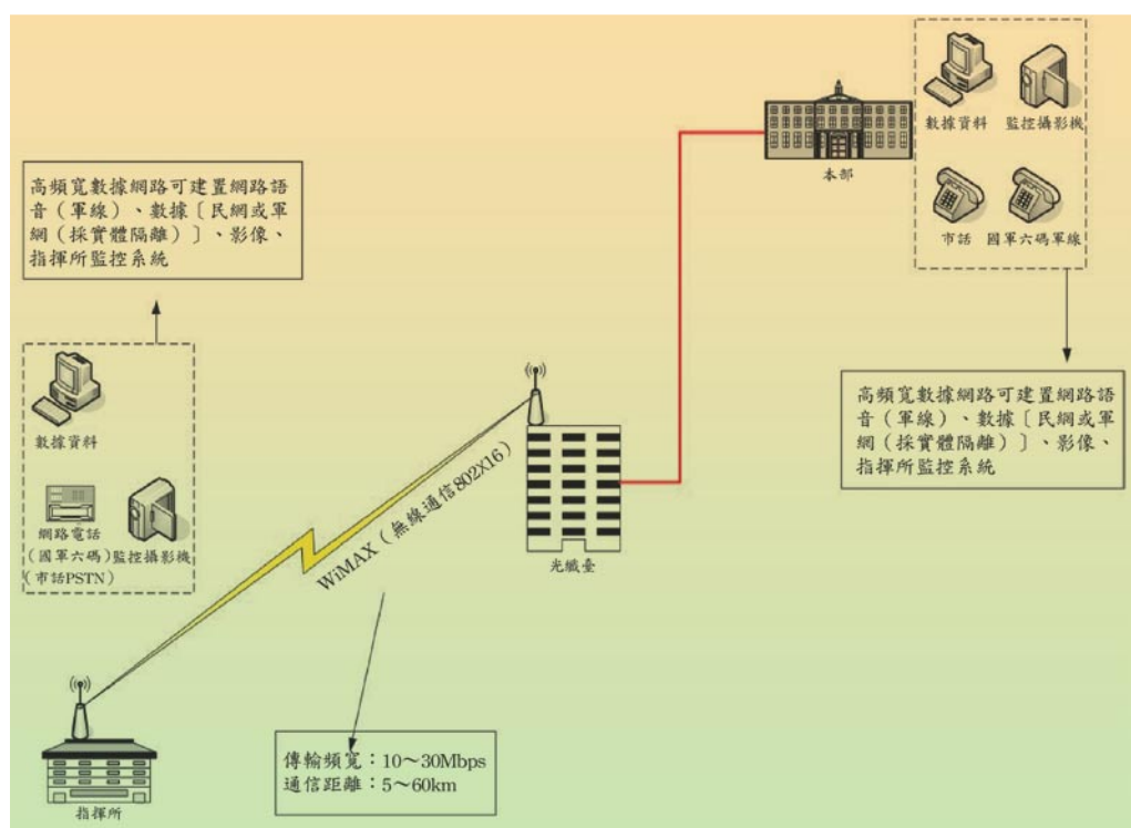
圖六 WiMAX結合光纖臺通信架構圖
