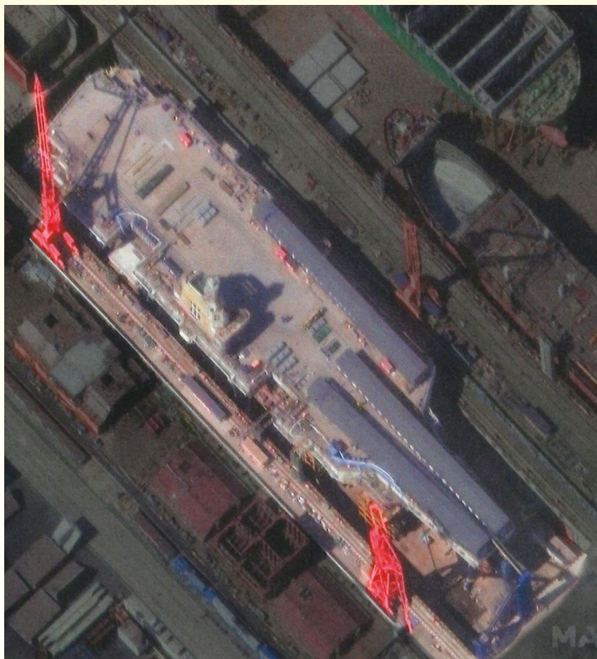
2022年2月在上海建造中的中共自製003型航空母艦衛星照片。其中值得注意之處在於用掩體覆蓋的，是該航艦規劃中的三具電磁發射彈射器。該艦建成後預計排水量為八萬噸。(Source: Maxar Technologies)
