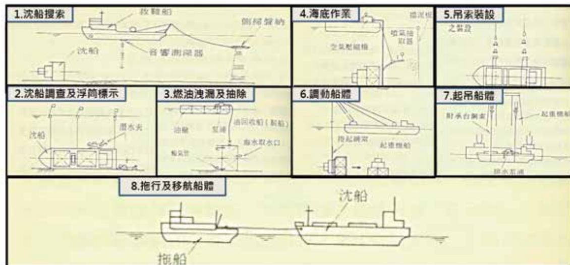
圖 10 沉船搜（撈）救作業程序
