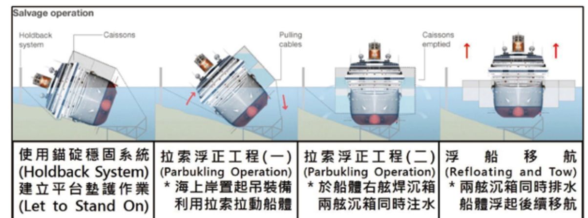
圖13 義大利歌詩達協和郵輪沉船救(撈)作業程序
