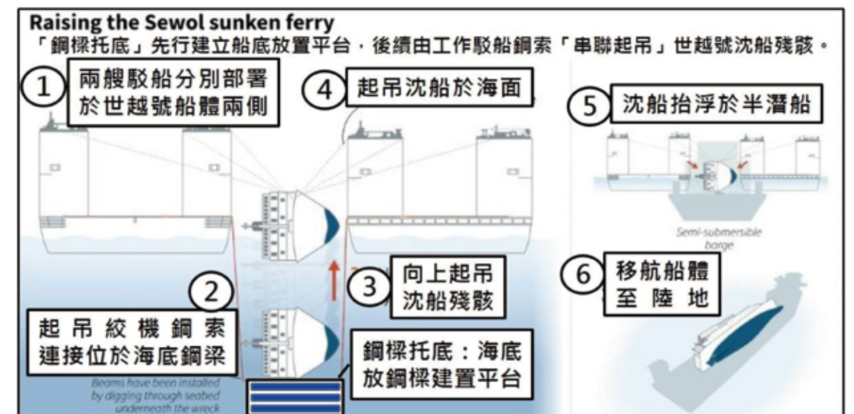
圖 15 南韓世越號沉船救 (撈) 作業程序
