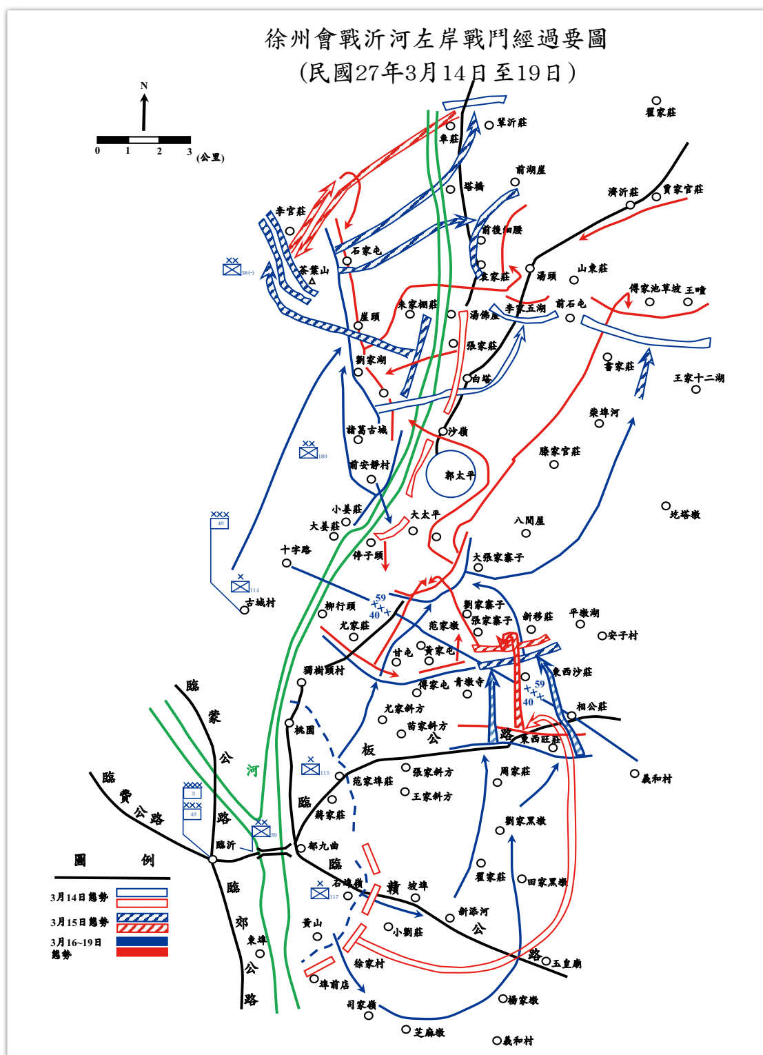
圖2 徐州會戰沂河左岸戰鬥經過要圖
