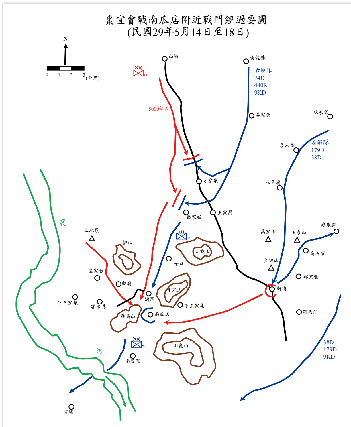
圖3 棗宜會戰南瓜店附近戰鬥經過要圖
