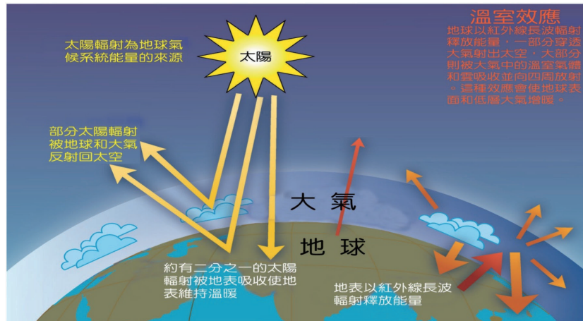
圖2 自然溫室氣體效應的理想模式
