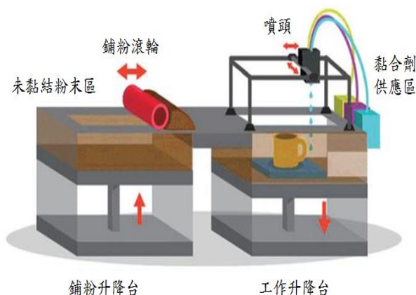
圖八：三維粉末黏接成型示意圖
