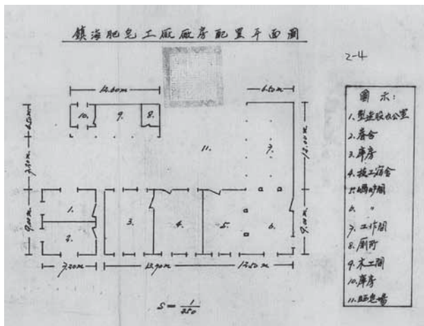
廠房配置平面圖
