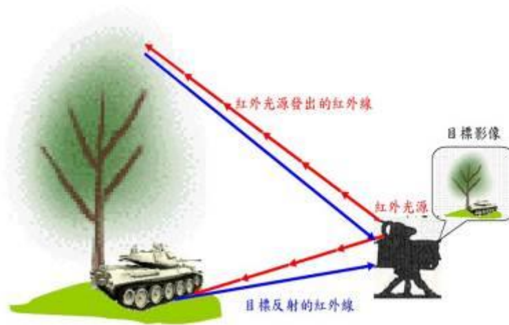
圖三 主動式紅外線夜視儀作用原理示意圖
