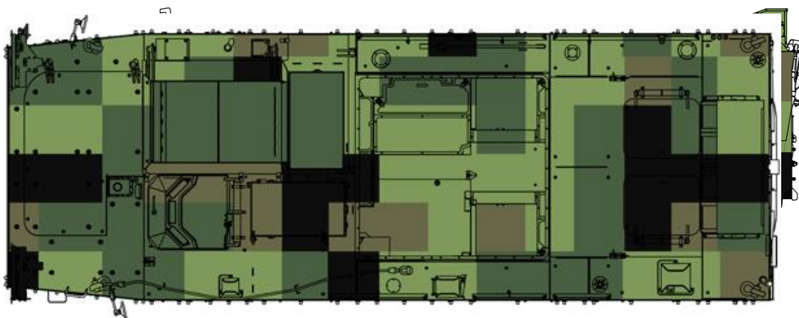
圖五 八輪甲車數位迷彩塗裝示意圖
