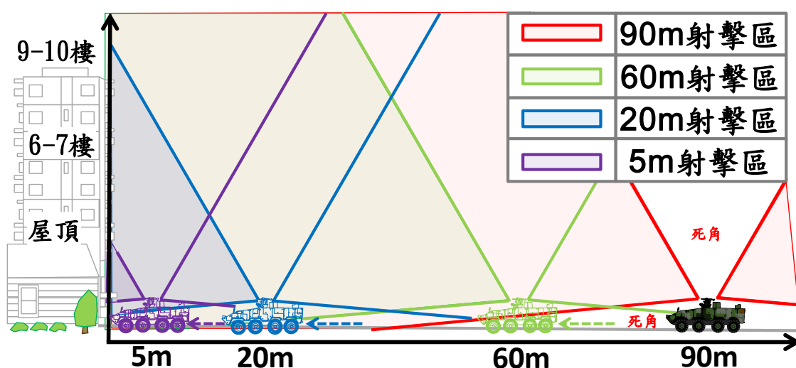
圖八：車裝武器射擊角度限制火力效果示意圖
