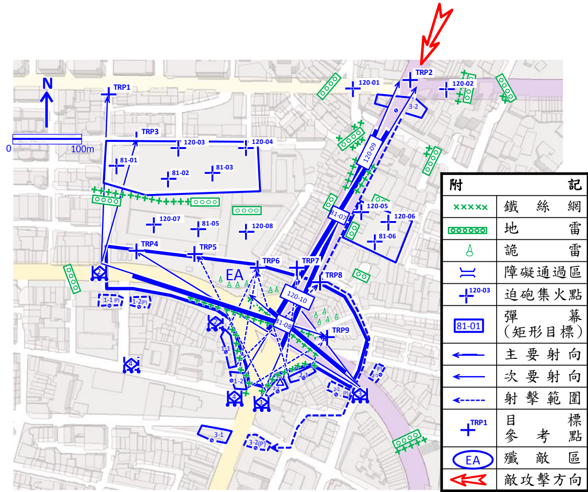
圖十一：機步排城鎮重要路口火力運用示意圖
