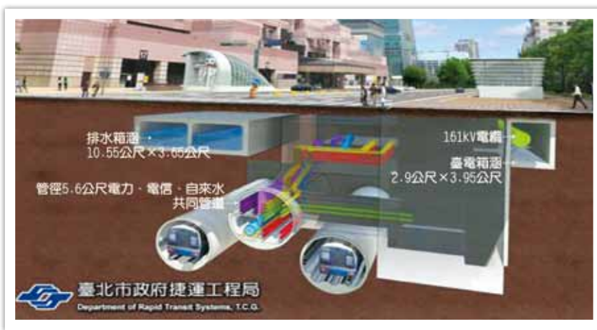
圖一 臺北市捷運、共同管道等地下設施透視圖
