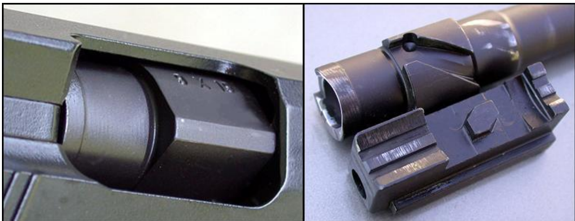
圖 5 PX4 Storm 槍管短後座、旋轉式閉鎖之外部特徵
