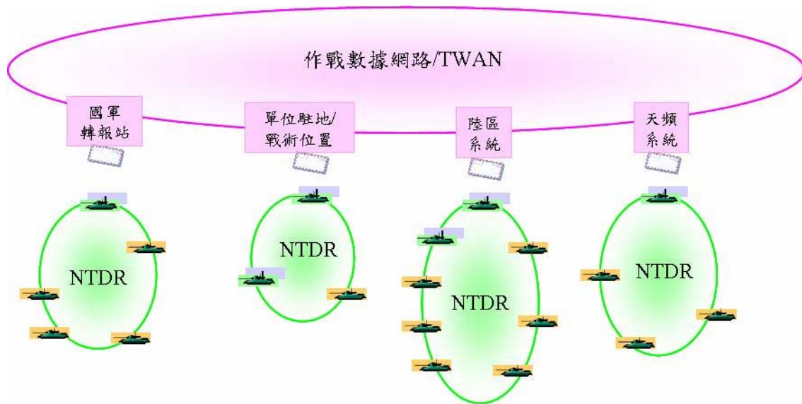
圖四 戰術訊號之擷取點架構示意圖(作者繪製)
