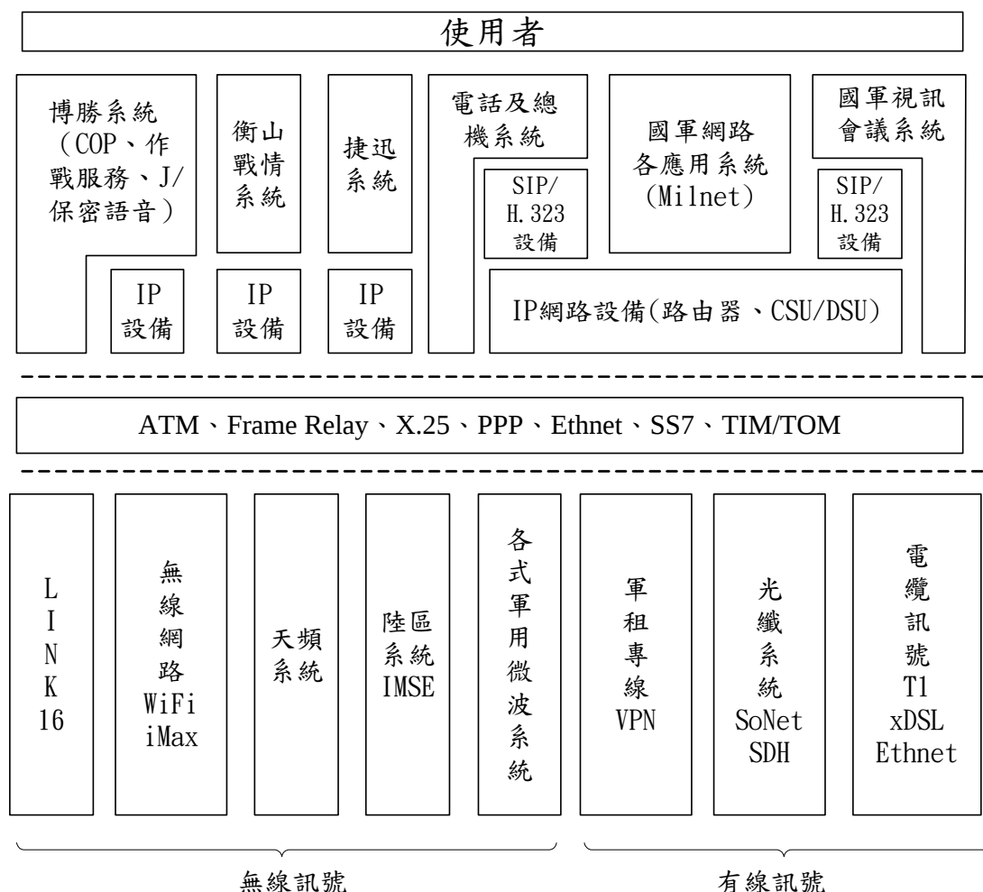
圖二 陸軍通資應用架構圖(作者繪製)
