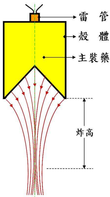
圖 1：錐形裝藥聚能效應示意圖
