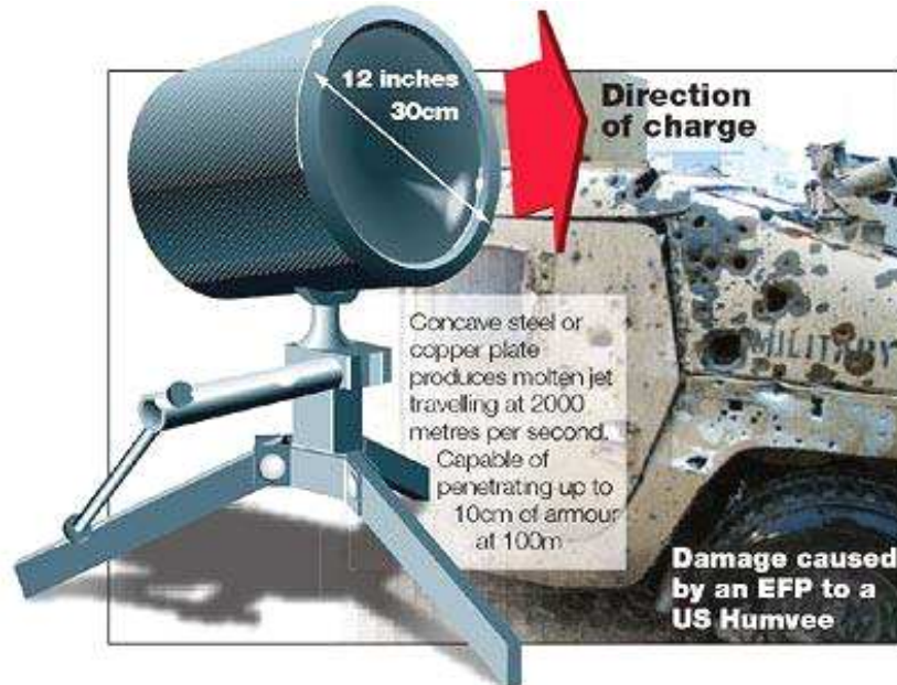
圖13：爆炸成形彈可於100公尺外穿透10公分厚的裝甲
