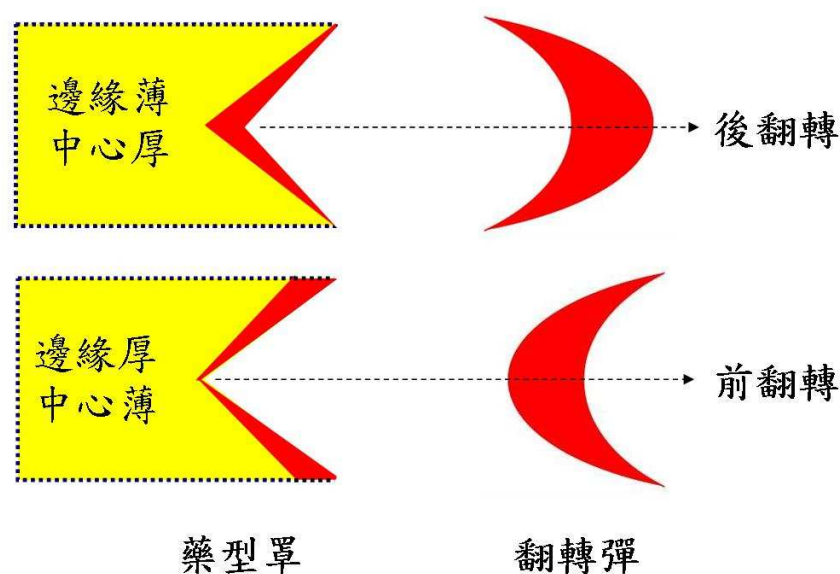
圖6：不同厚度藥型罩形成不同形狀之翻轉彈示意圖
