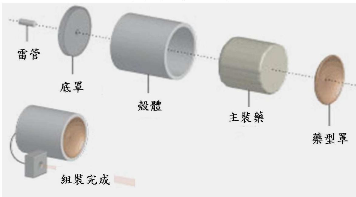
圖3：爆炸成形彈的組成示意圖
