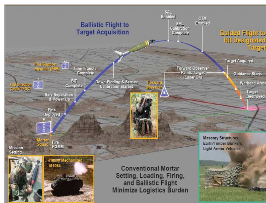
圖 9：美國精確導引迫擊砲彈 X935 導引流程圖 22
