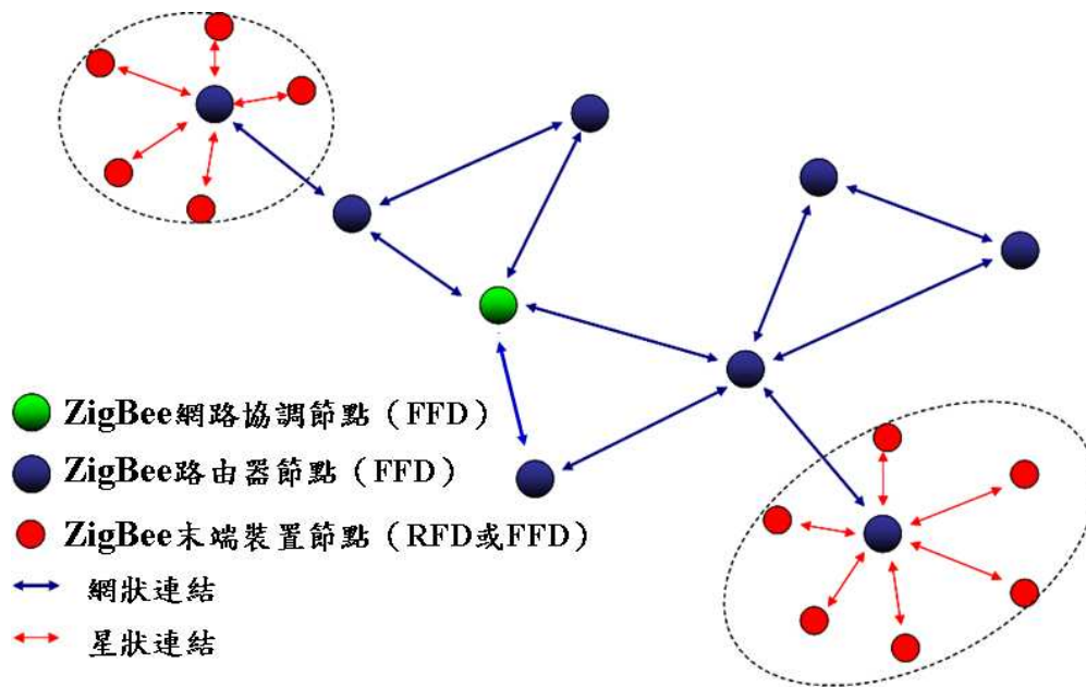
圖 3：ZigBee 網路架構
