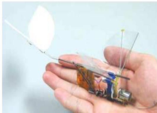
圖十 「微型蝙蝠」飛行器重 14 公克
